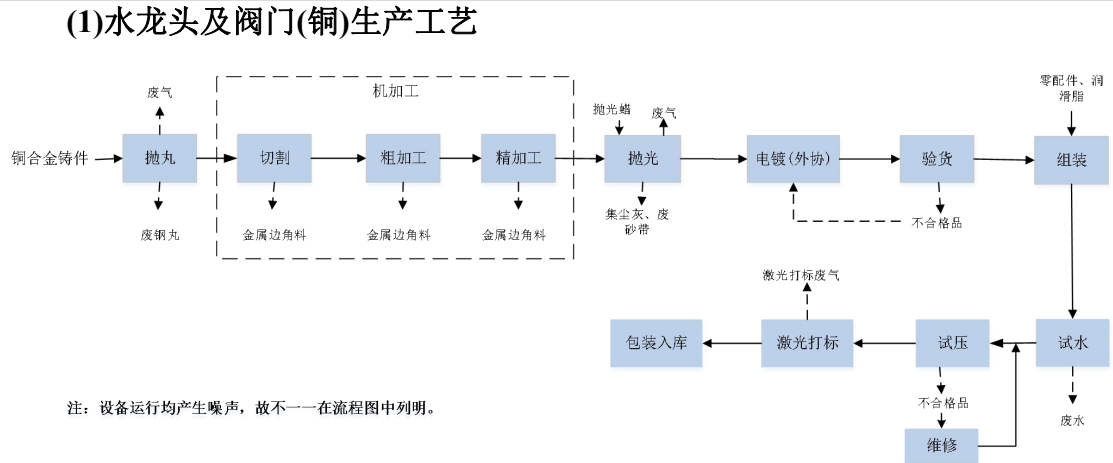
图 2-2 水龙头及阀门(铜)生产工艺及产污流程图
