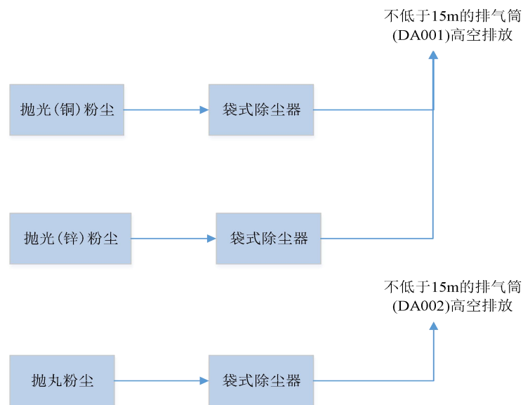
图 4-1 本项目废气处理方式
