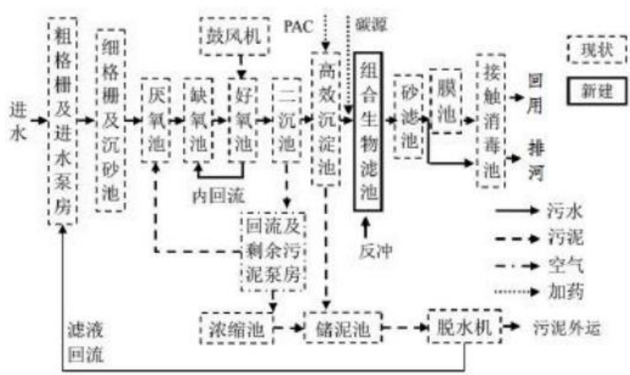
图 4-3 路桥污水处理厂废水处理工艺流程示意图
