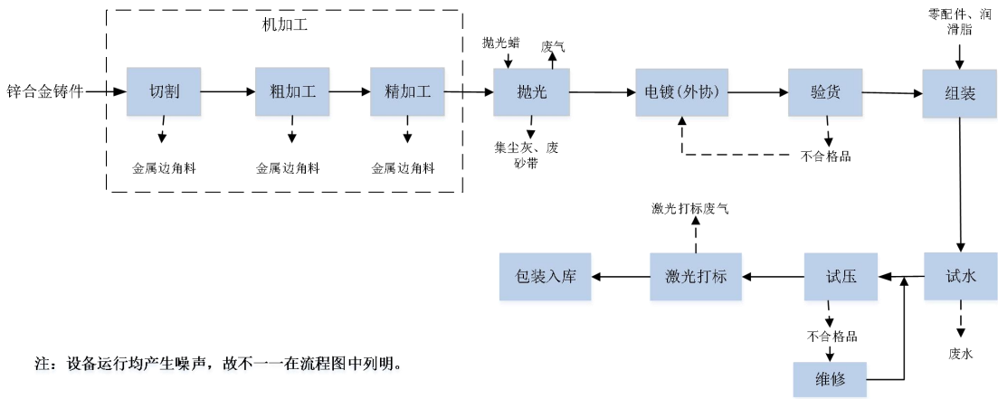
图 2-3 水龙头及阀门(锌)生产工艺及产污流程图
